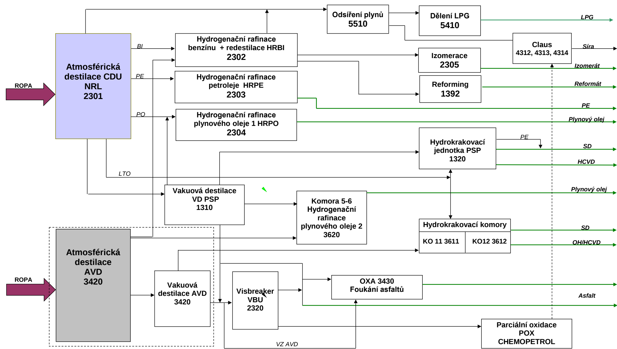
Zjednodušené schéma návaznosti provozních souborů - Destilace (LITVÍNOV)
